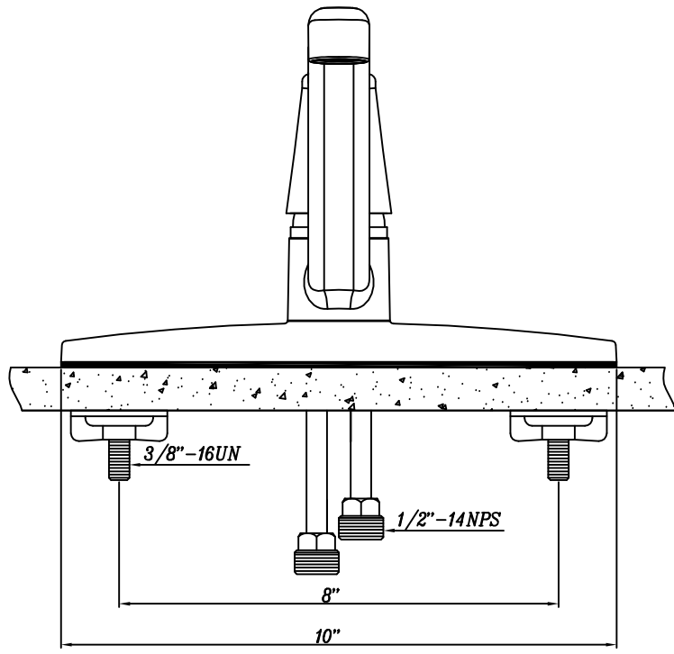
ESCUTCHEON LENGTH
