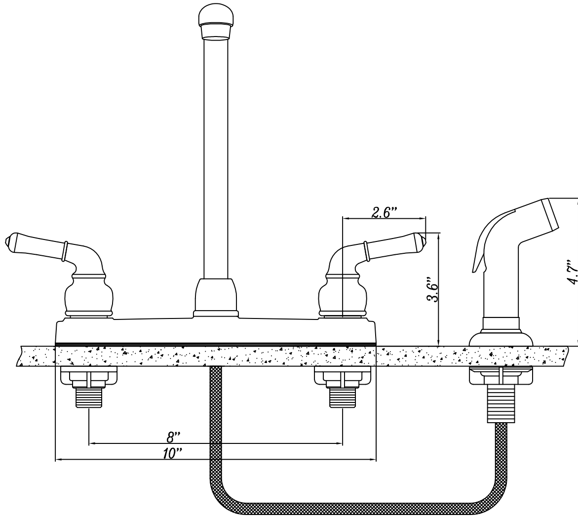
ESCUTCHEON LENGTH
