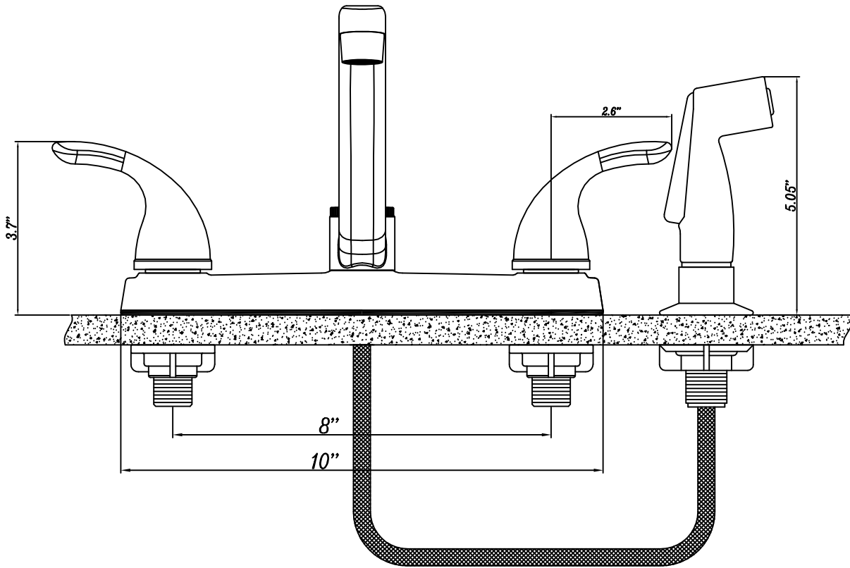
ESCUTCHEON LENGTH
