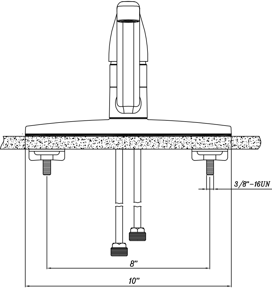
ESCUTCHEON LENGTH
