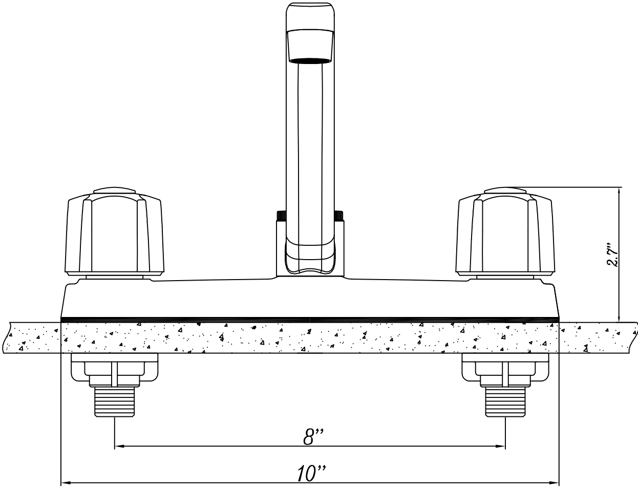
ESCUTCHEON LENGTH
