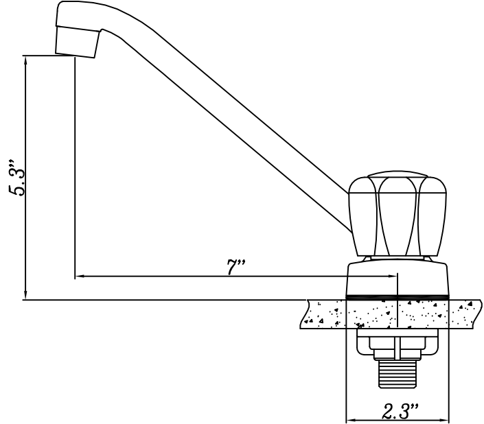
ESC. WIDTH
