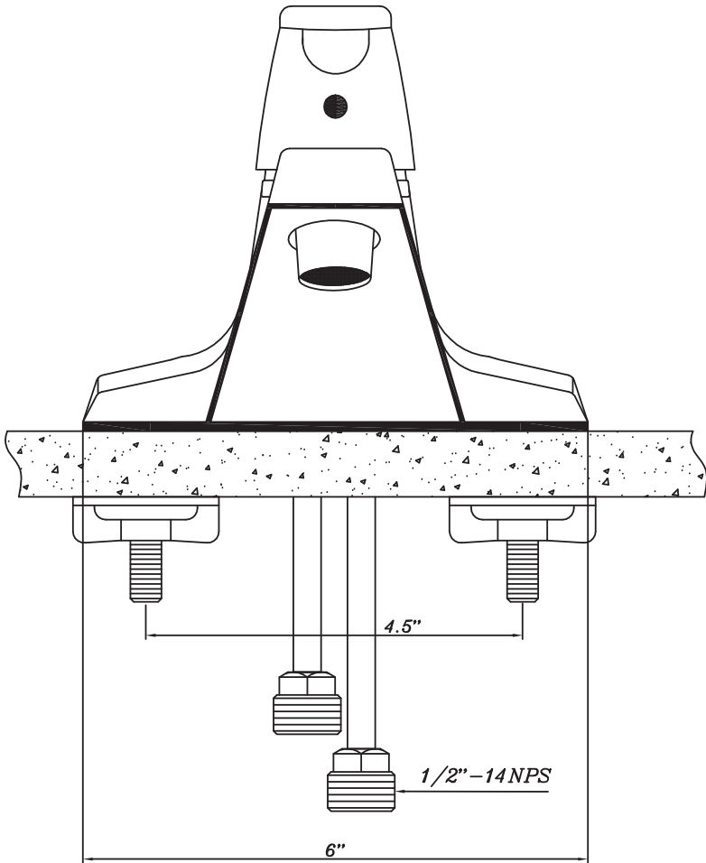
ESCUTCHEON LENGTH
