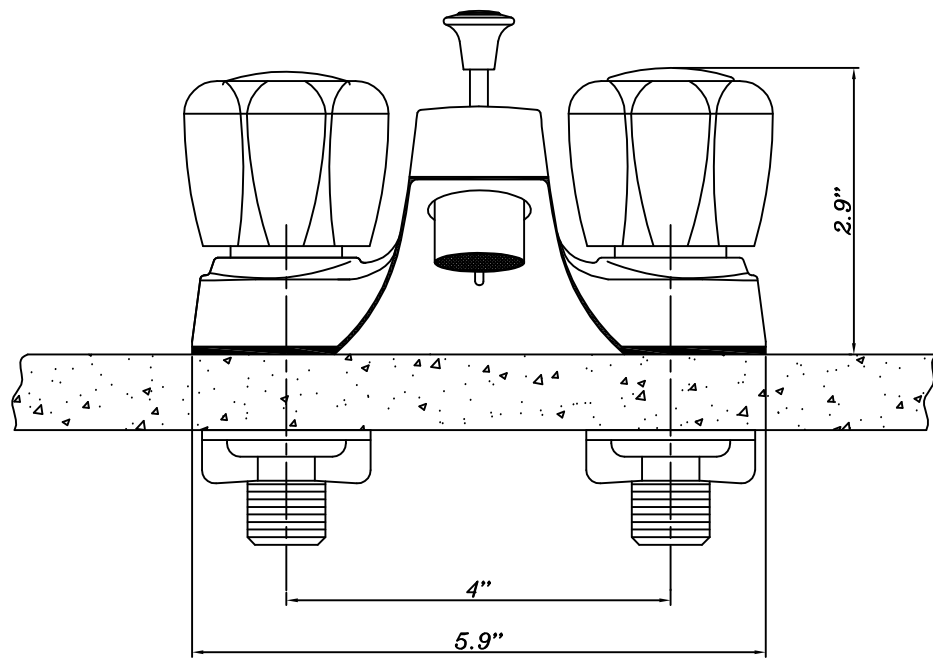
ESCUTCHEON LENGTH
